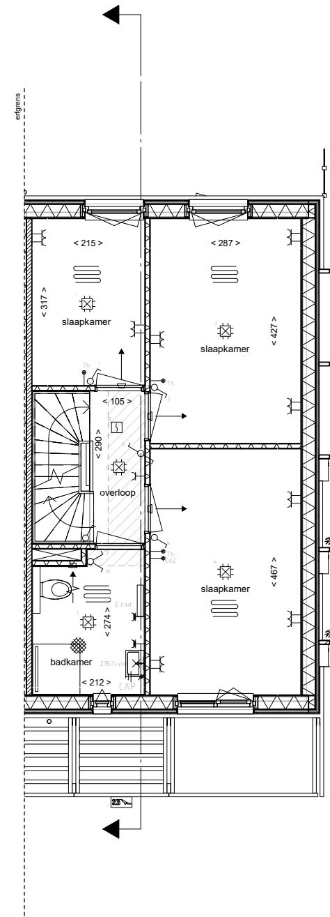
eerste verdieping
